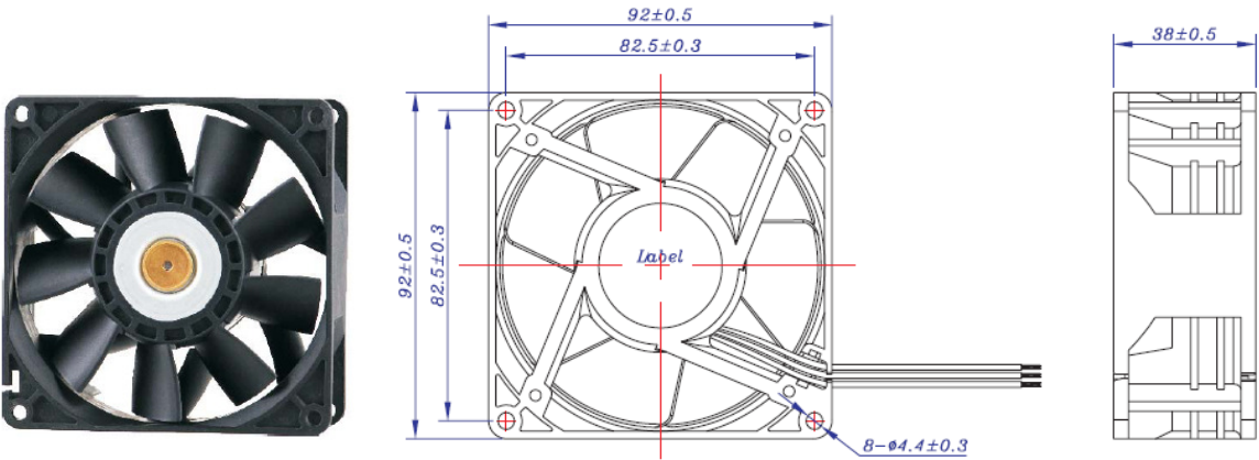
OUTLINE(mm)
