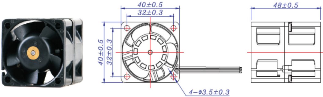
OUTLINE(mm)
