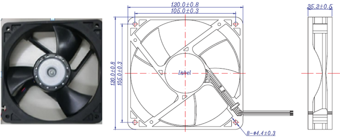
OUTLINE(mm)
